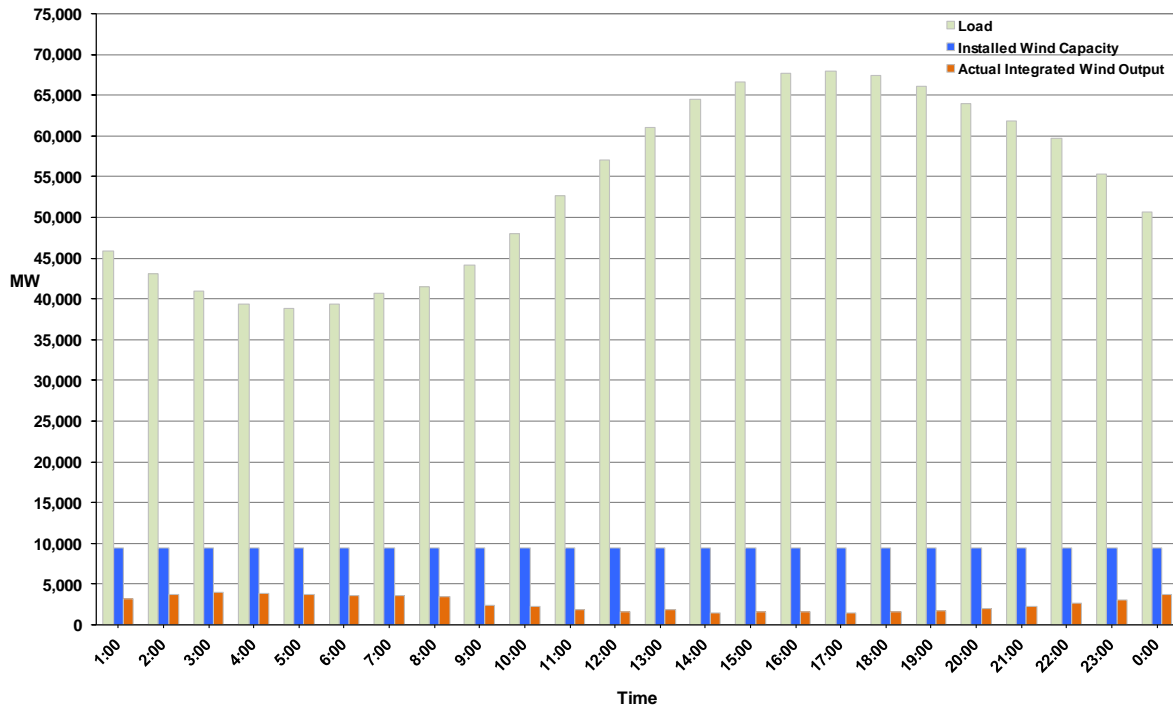
Hourly Average Actual Load vs. Actual Wind Output 08-02-2011
