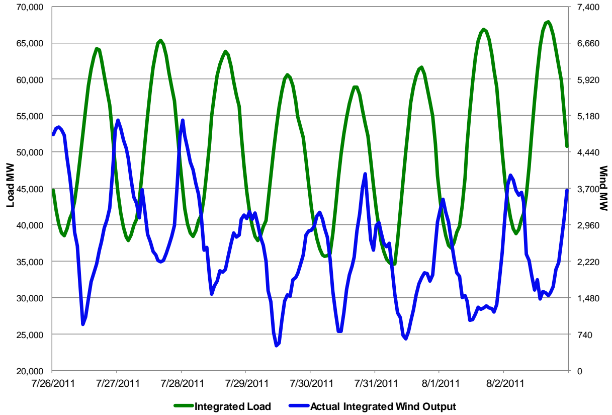
ERCOT Load vs. Actual Wind Output 7/26/2011 - 8/2/2011
